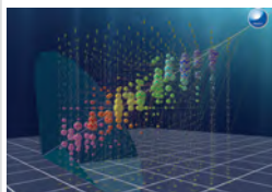
interazione di neutrini
