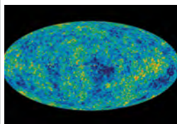
radiazione cosmica di fondo
