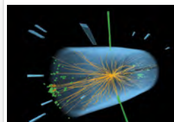
collisioni ad alta energia
