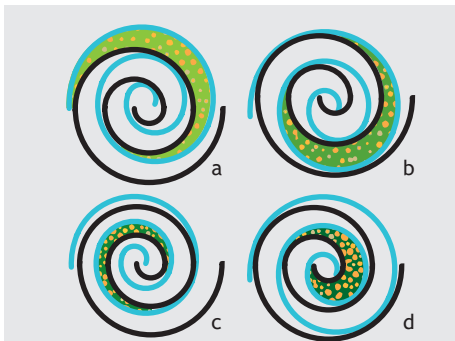
spirale fissa e spirale mobile
