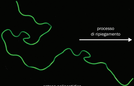
catena polipeptidica
