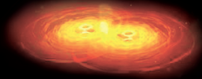
buchi neri supermassivi
